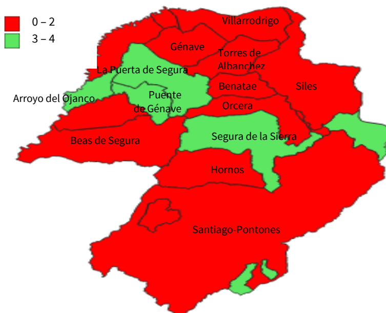
Mapa. Consumo de energía eléctrica por habitante, 2022
