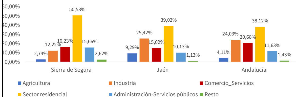
Gráfico. Consumo de energía eléctrica por sectores económicos 2022 (%)
