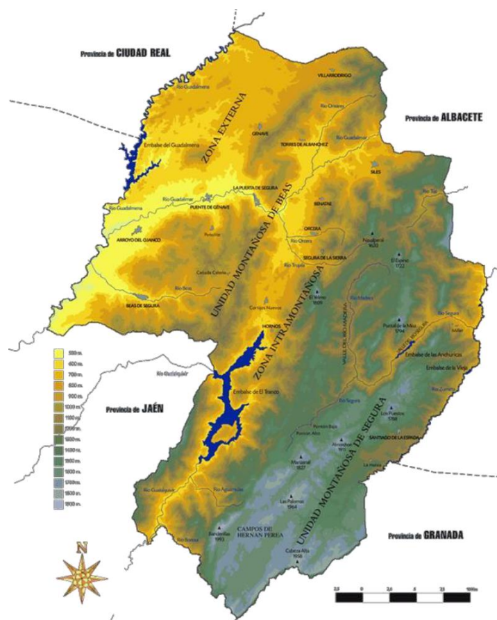
Figura 1. Orografía de Sierra de Segura
